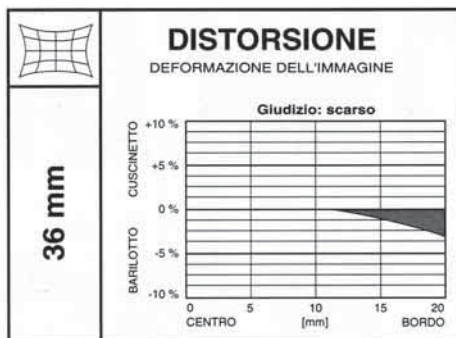
▲ Figura 3 - Distorsione a barilotto
