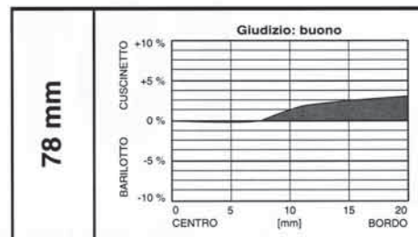
▲ Figura 4 - Distorsione a cuscinetto
